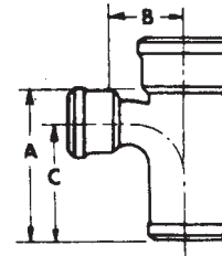
FIG. 36 Straight Tees
