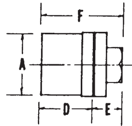
FIG. 24 Pipe Plugs
