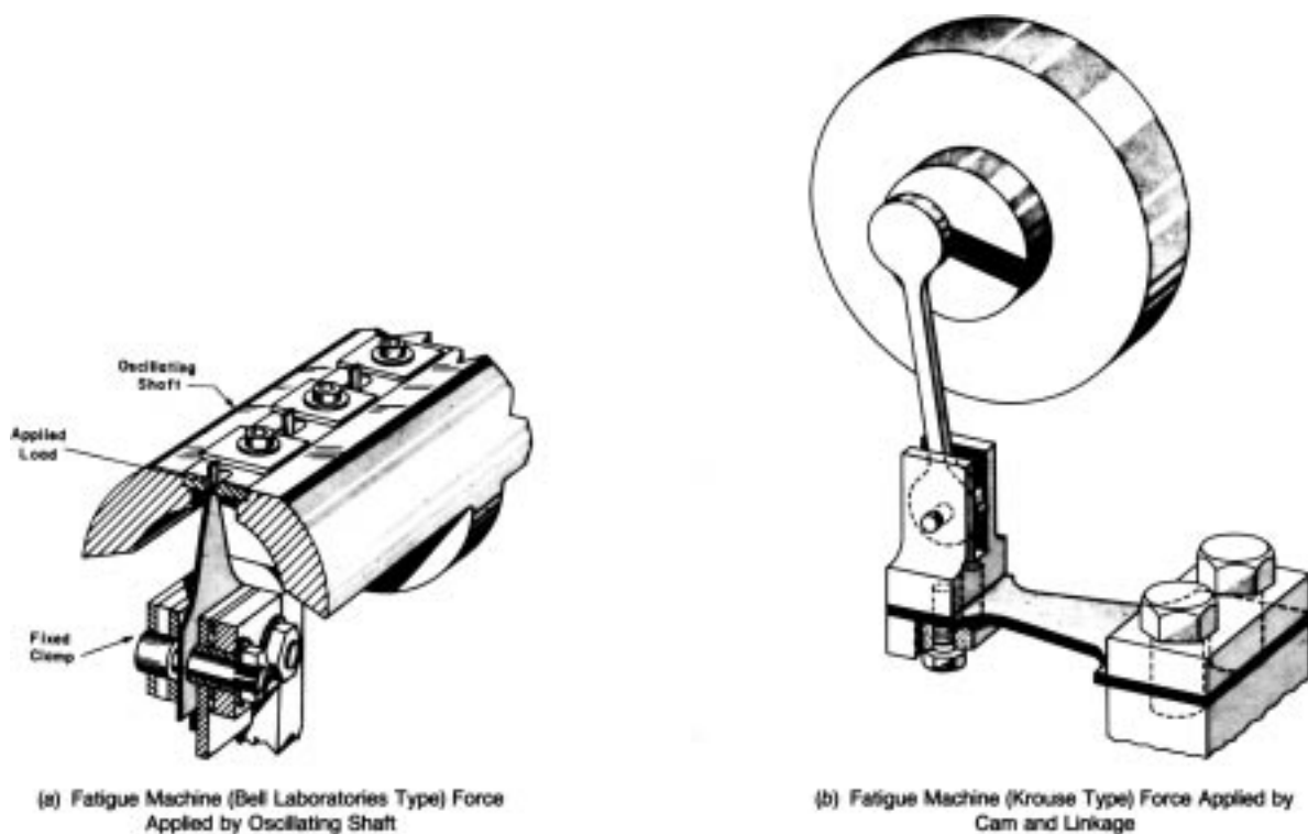
FIG. 1 Fatigue Machines
