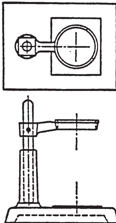
FIG. 2 Stand
