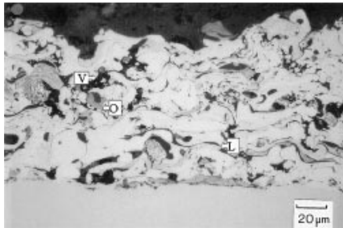
FIG. 8 Ni/Al TSC—500X
