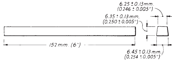
FIG. 3 Izod Impact Test Bar for Die Castings Alloys
