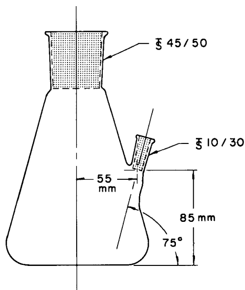
FIG. X1.2 Modified Erlenmeyer Flask (1000 mL)
