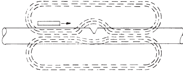
FIG. 4 Longitudinal Magnetization
