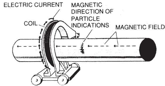
FIG. 11 Longitudinal Magnetization
