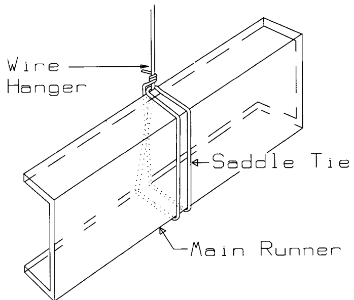
FIG. 3 Saddle-Tie
