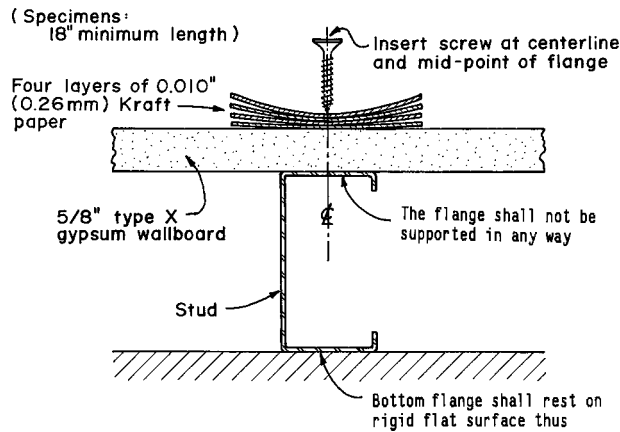
FIG. 3 4 Studs
