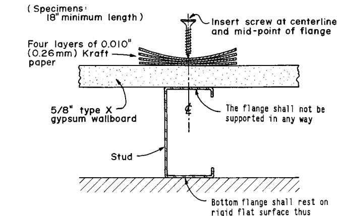
FIG. 1 Studs
