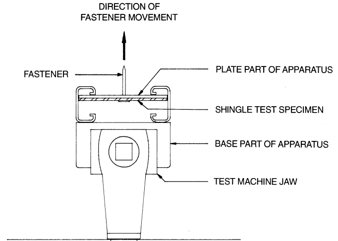
FIG. 2 Apparatus
