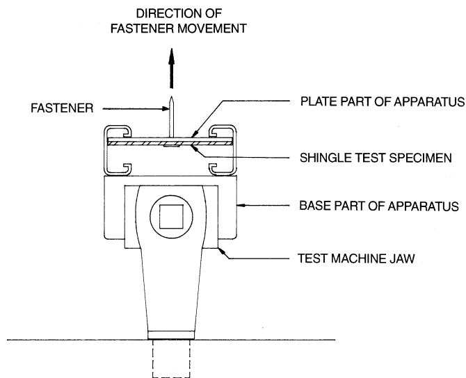
FIG. 2 Apparatus
