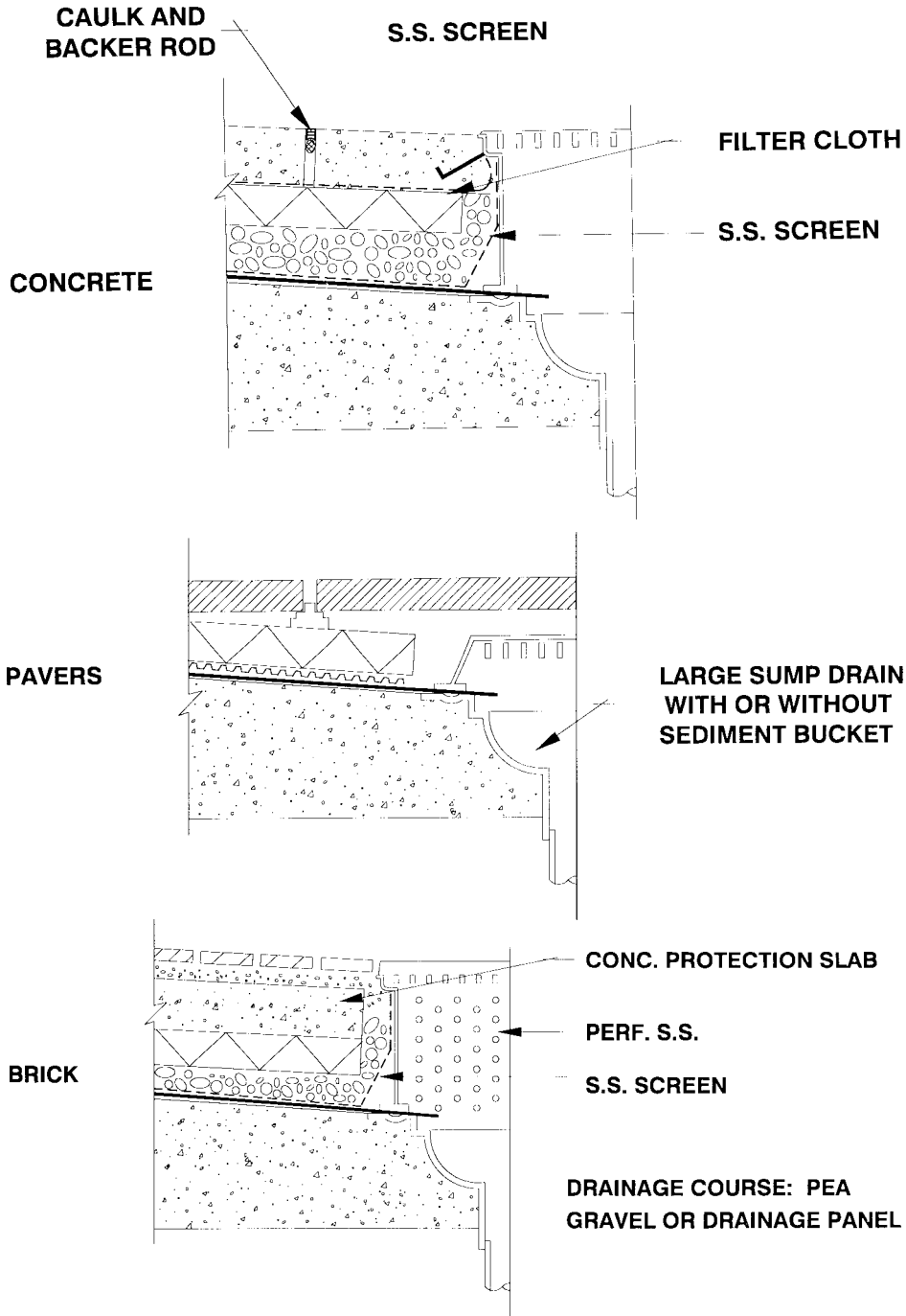
FIG. 20 Drain
