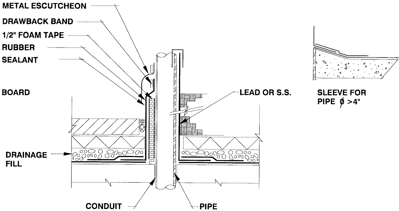
FIG. 18 Pipe/Conduit Penetration
