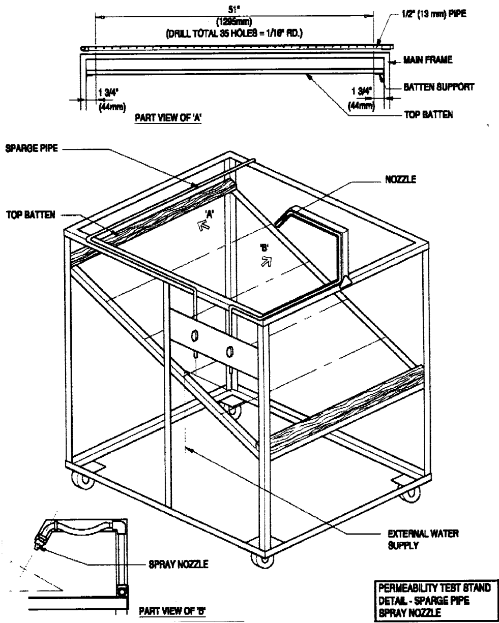
FIG. 3 Diluge Pipe
