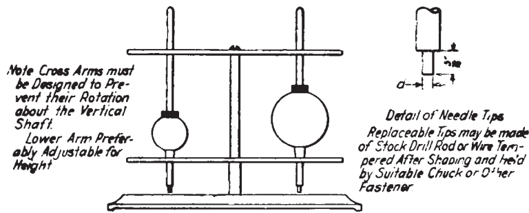
FIG. 1 Gilmore Apparatus
