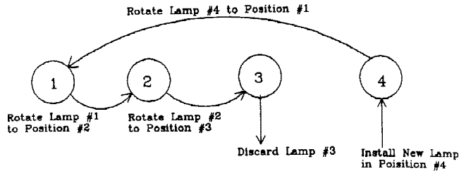
FIG. 4 UV Lamp Rotation
