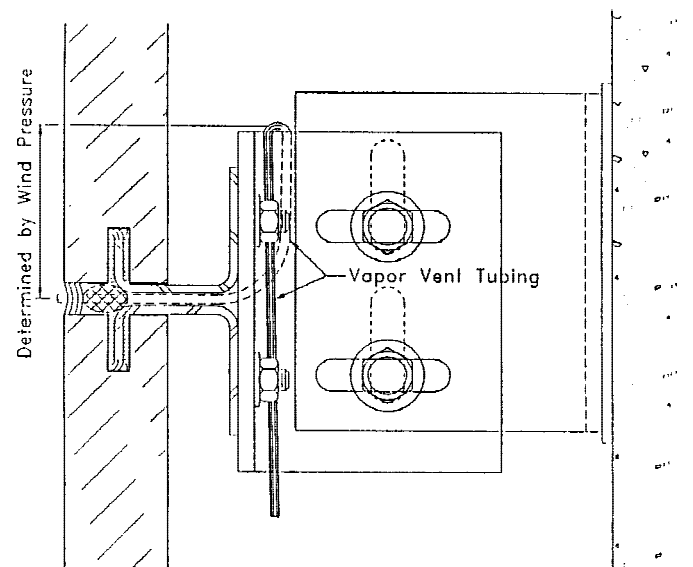
FIG. 11 Vapor Vent Tubing
