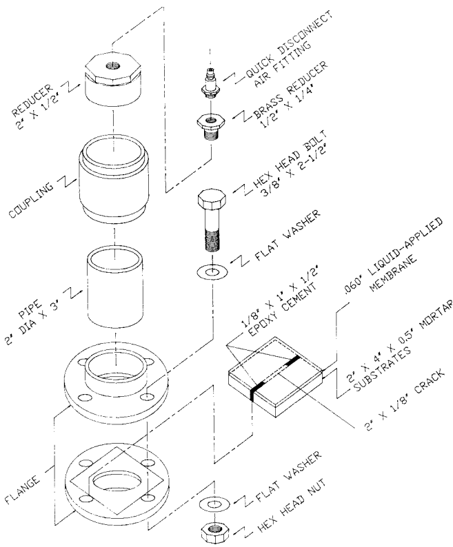
FIG. 1 Testing Apparatus
