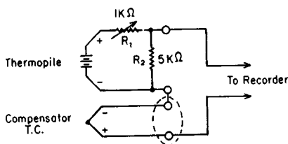
FIG. 12 Wiring Diagram
