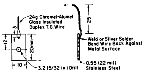
FIG. 10 Compensator Tab
