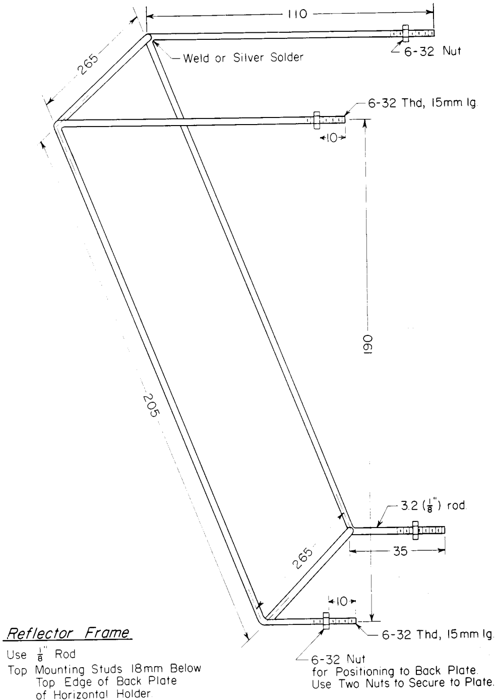
FIG. 21 Reflector Frame
