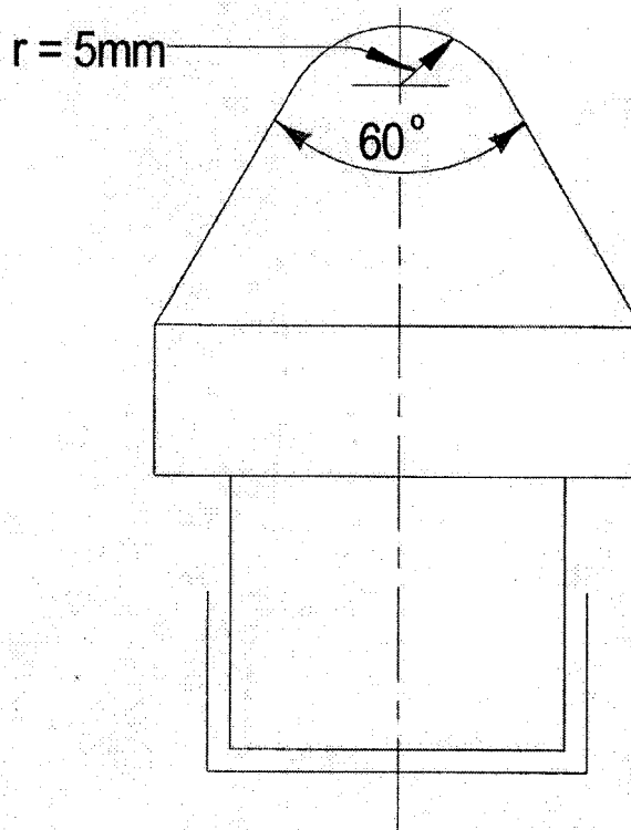
FIG. 2 Platen Dimensions
