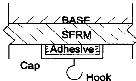
FIG. 2 In-Place Apparatus
