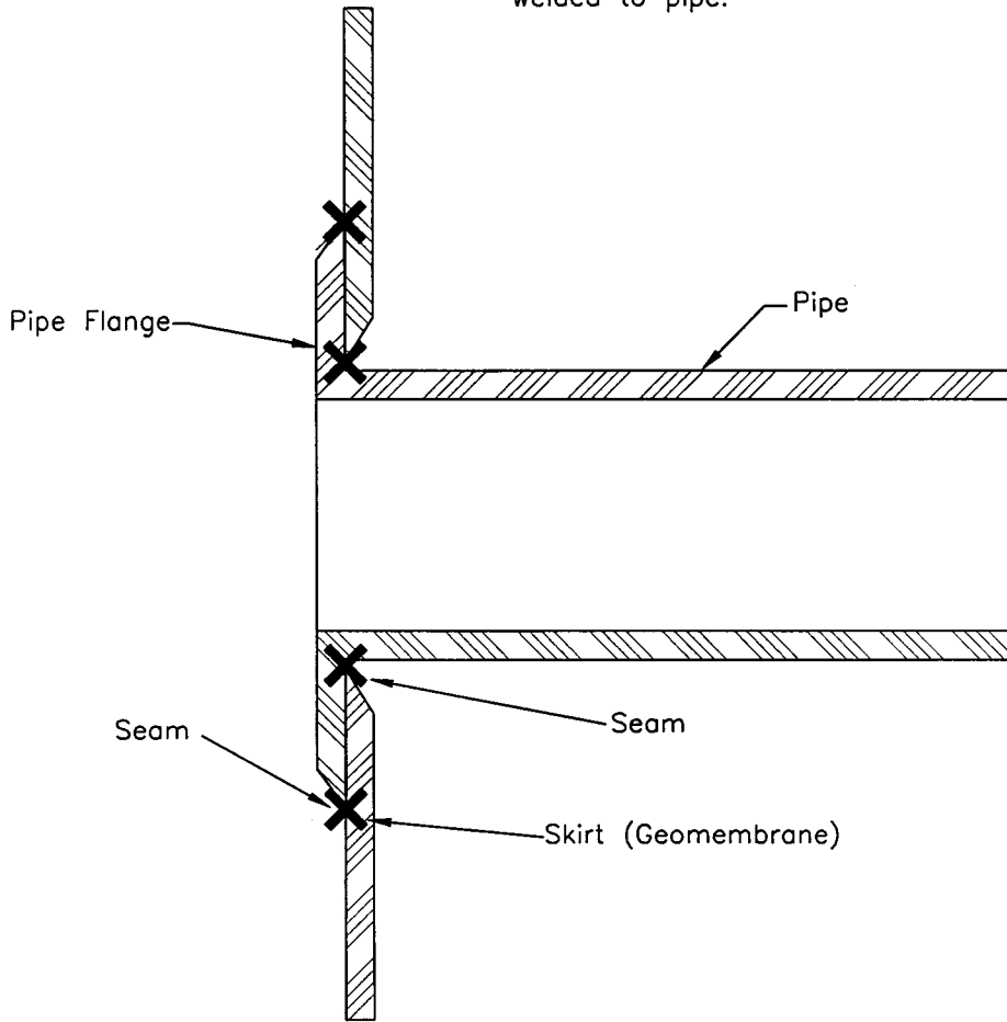
FIG. 13 Pipe Boot
