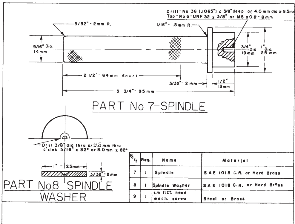
FIG. 4 Spindle
