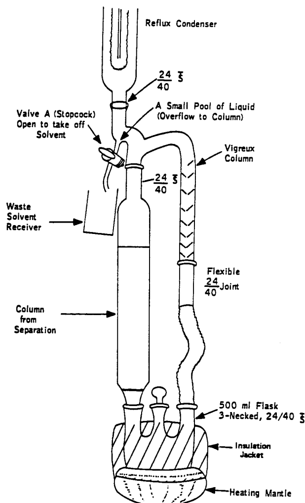
FIG. 3 Extraction Apparatus
