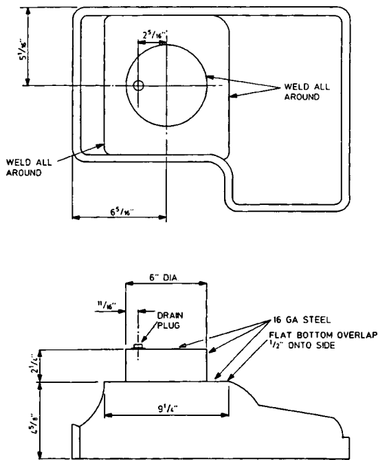
FIG. A3.24 Camshaft Baffle Fabrication
