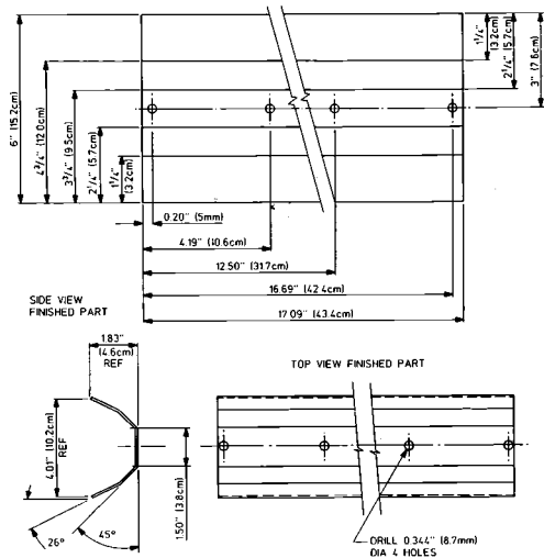
FIG. A3.24 Camshaft Baffle Fabrication
