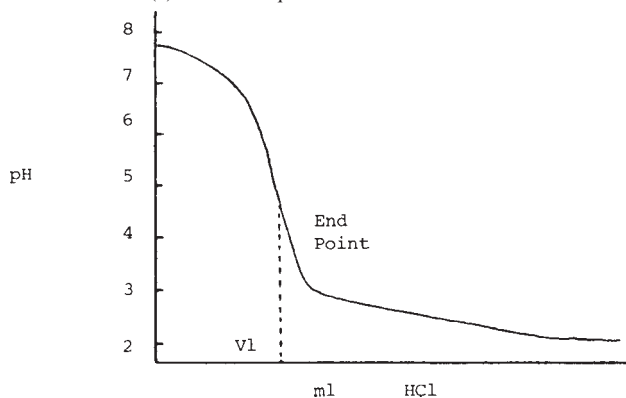
(b) Base Milliequivalent Content Titration
