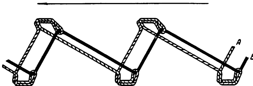
FIG. 23 Stitch Type 313
