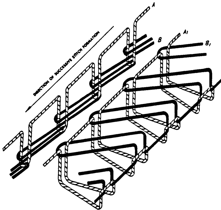
FIG. 47 Stitch Type 514
