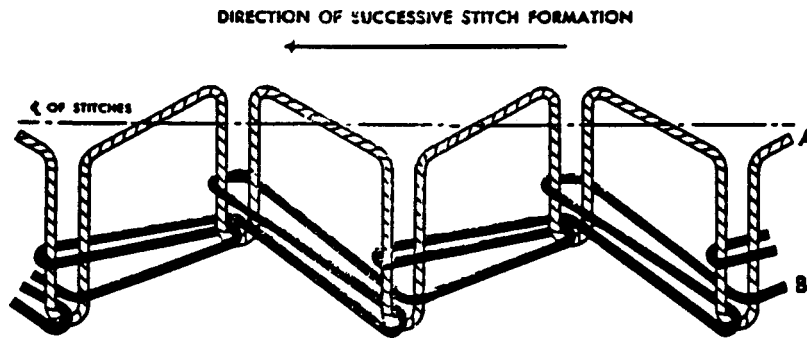
FIG. 30 Stitch Type 404
