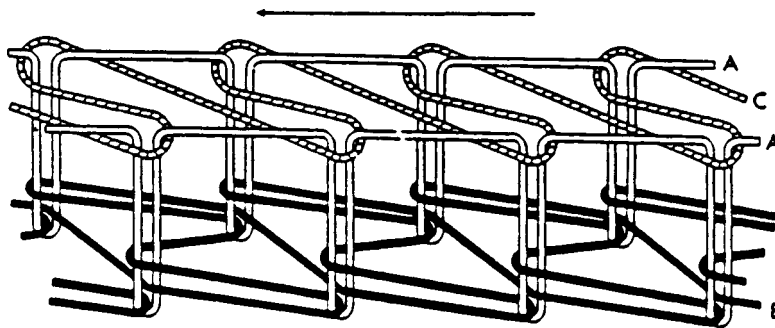
FIG. 56 Stitch Type 601
