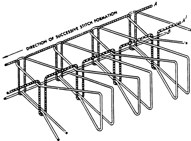
FIG. 41 Stitch Type 508
