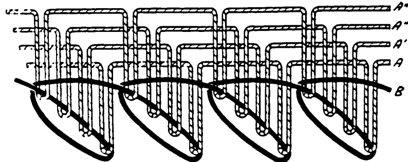
FIG. 17 Stitch Type 307
