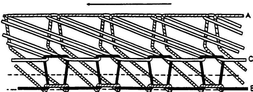
FIG. 37 Stitch Type 504
