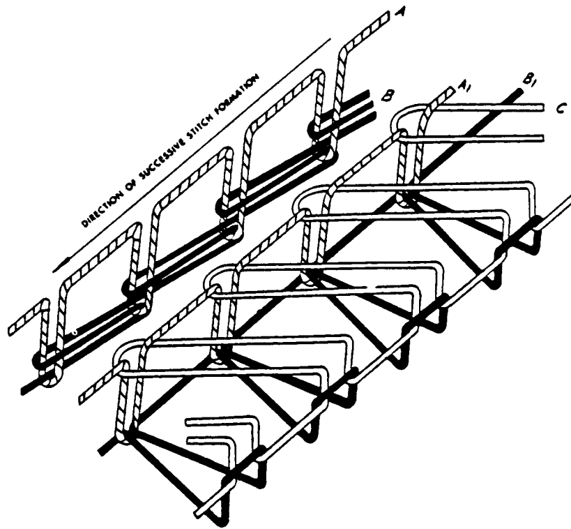
FIG. 49 Stitch Type 516
