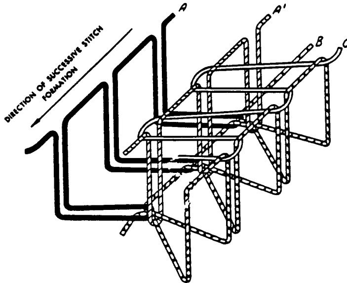
FIG. 39 Stitch Type 506
