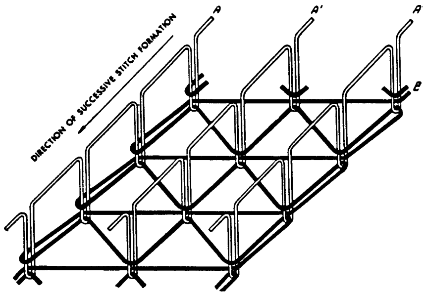
FIG. 33 Stitch Type 407
