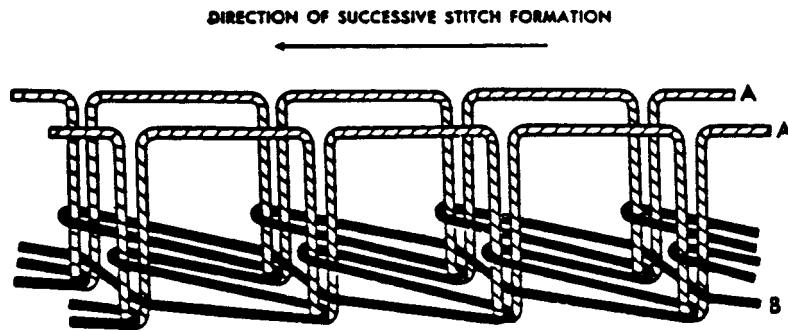
FIG. 31 Stitch Type 405
