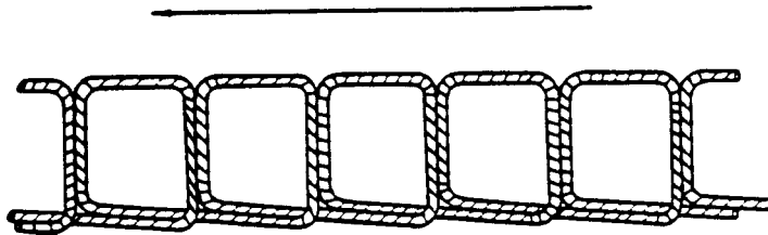
FIG. 7 Stitch Type 202
