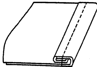
Seam type SSp-1
