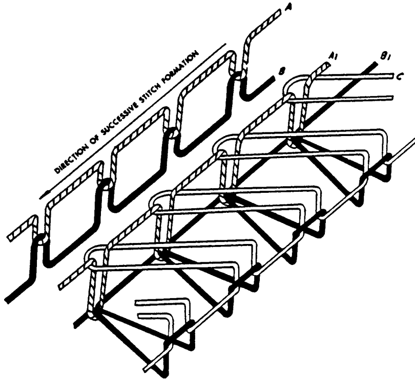
FIG. 50 Stitch Type 517
