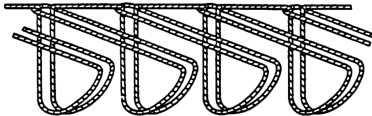
FIG. 3 Stitch Type 103
