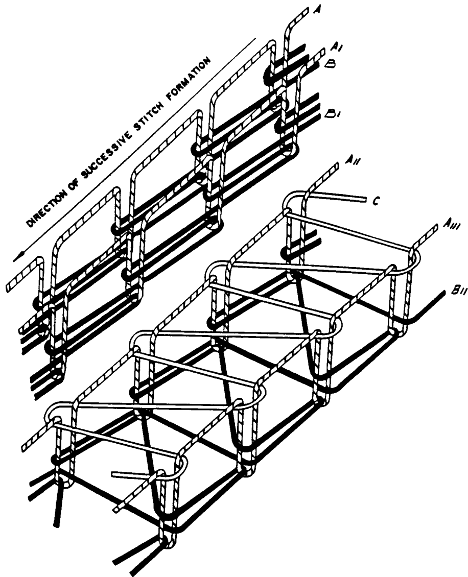
FIG. 53 Stitch Type 520
