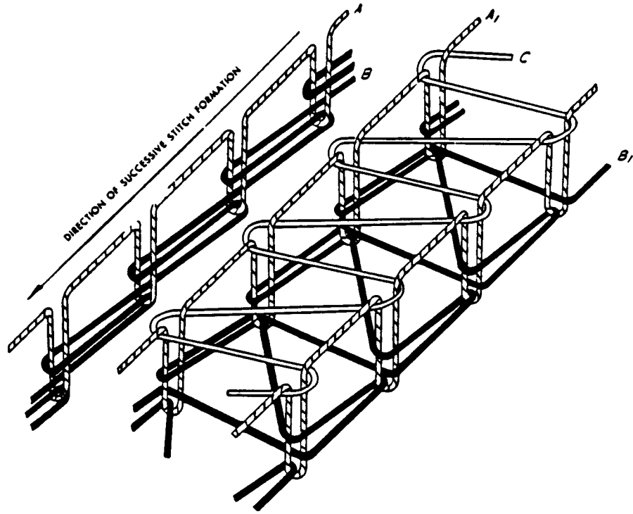
FIG. 52 Stitch Type 519
