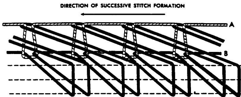
FIG. 34 Stitch Type 501
