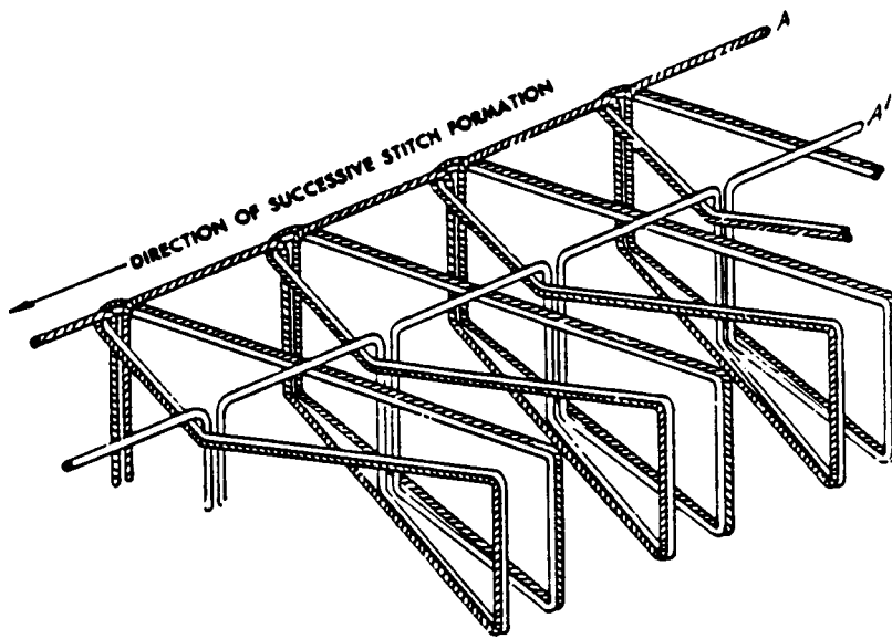
FIG. 43 Stitch Type 510
