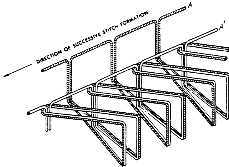
FIG. 43 Stitch Type 510
