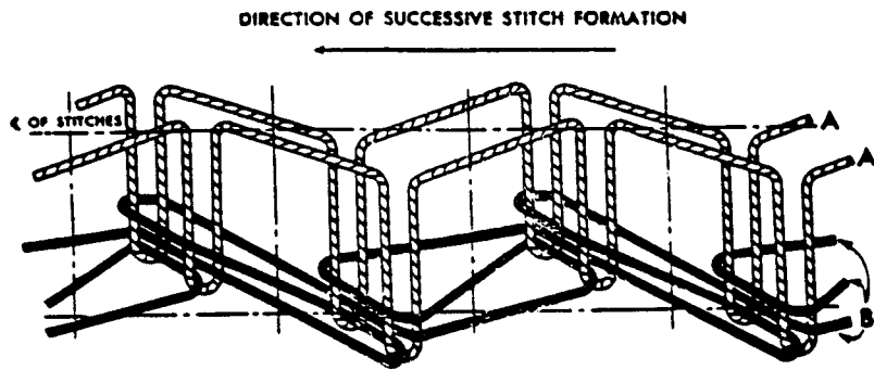
FIG. 30 Stitch Type 404
