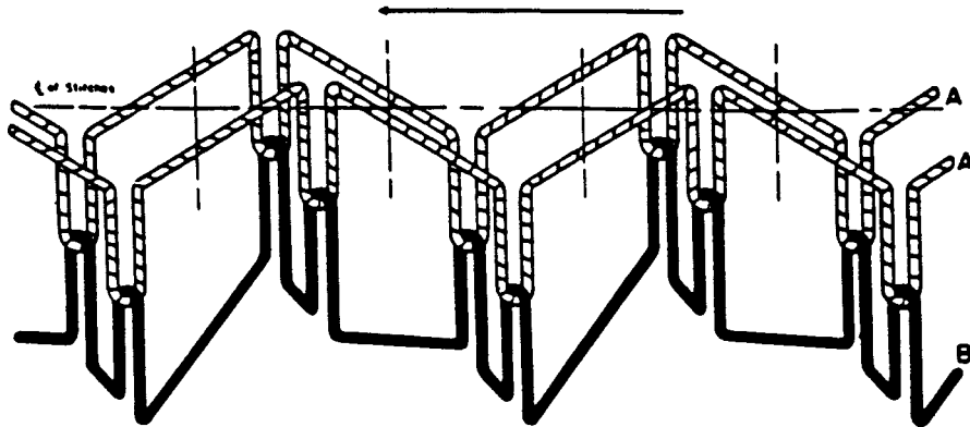
FIG. 22 Stitch Type 312
