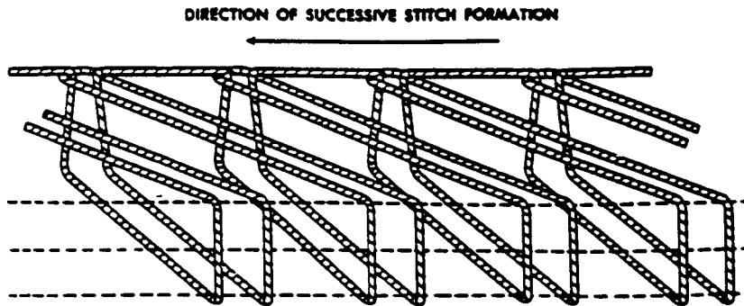
FIG. 33 Stitch Type 407
