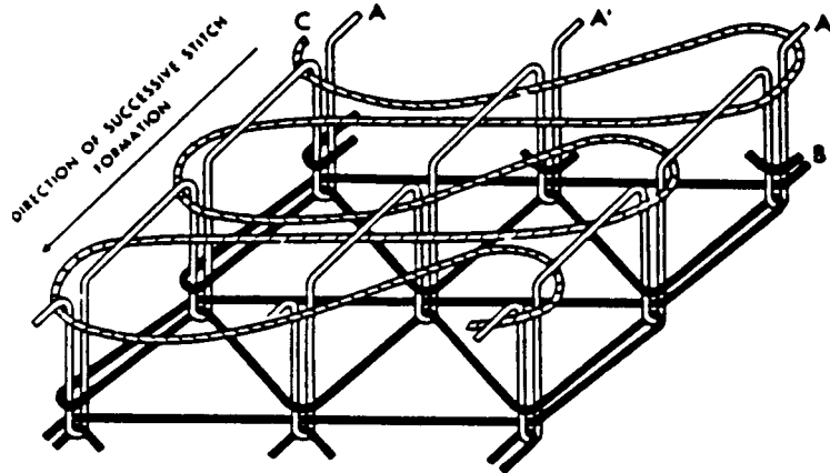
FIG. 59 Stitch Type 604
