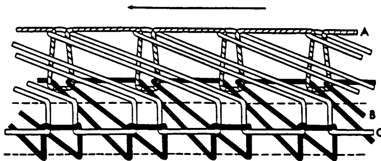
FIG. 36 Stitch Type 503
