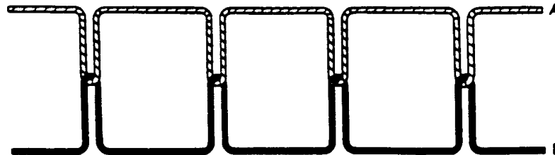
FIG. 10 Stitch Type 205
