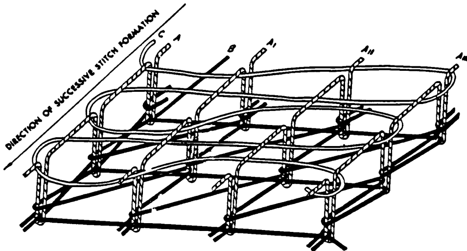
FIG. 61 Stitch Type 606
