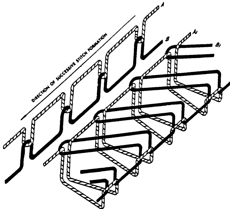
FIG. 50 Stitch Type 517
