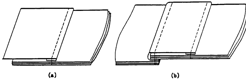
FIG. 212 Seam Type LScy-3
