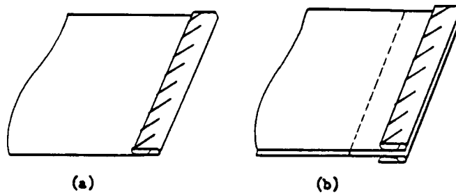
FIG. 108 Seam Type SSaz-1
