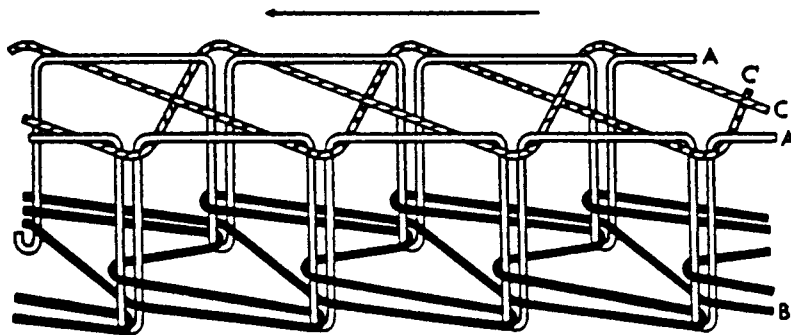
FIG. 57 Stitch Type 602
