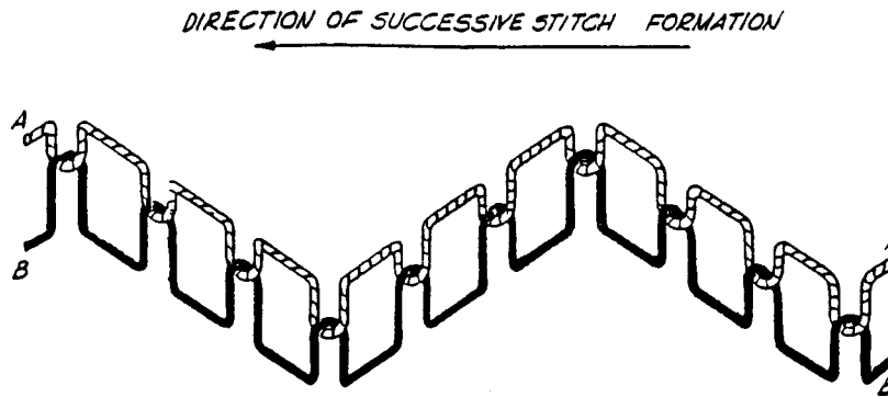
FIG. 24 Stitch Type 314
