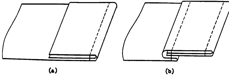
FIG. 216 Seam Type LSdc-3
