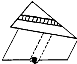
FIG. 242 Stitching Type O3a
