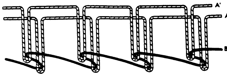
FIG. 19 Stitch Type 309
