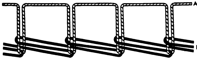
FIG. 27 Stitch Type 401
