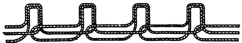
FIG. 4 Stitch Type 104
