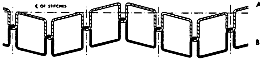
FIG. 18 Stitch Type 308
