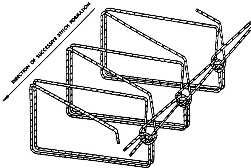
FIG. 45 Stitch Type 512
