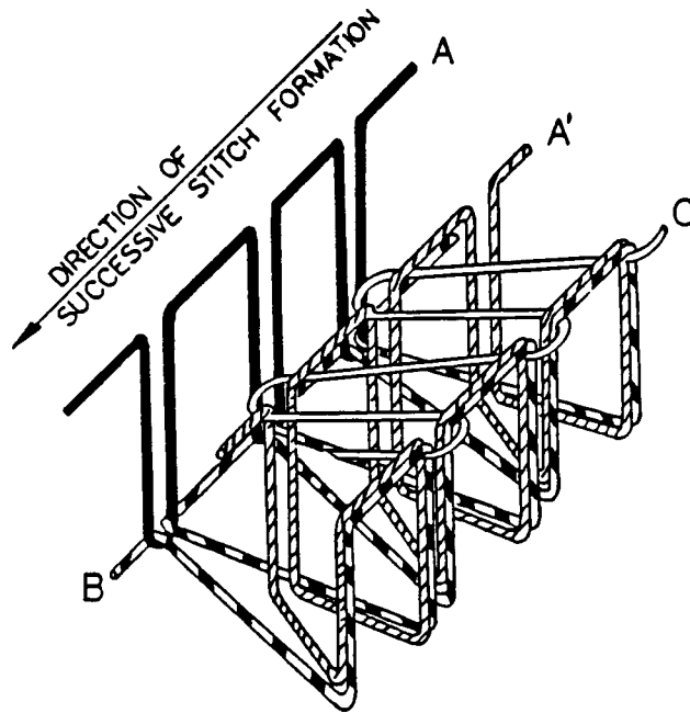
FIG. 54 Stitch Type 521
