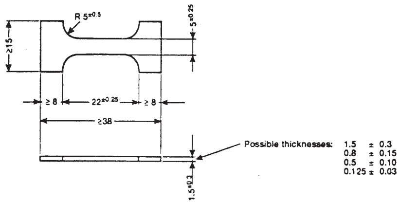
FIG. 11 Microtensile Die
