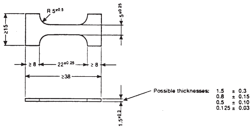
FIG. 11 Microtensile Die
