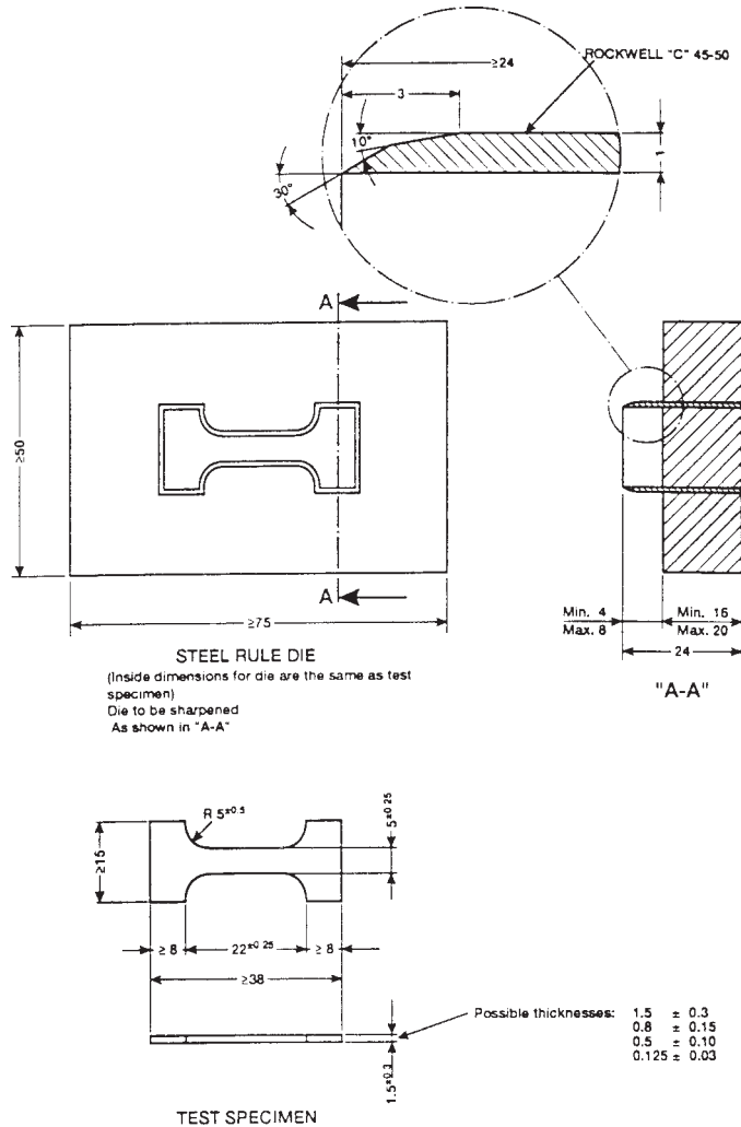
FIG. 8 Microtensile Die
