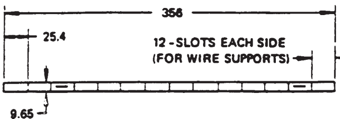
FIG. 5 Bottom U-Frame
