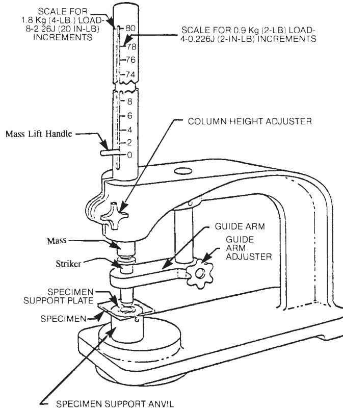
FIG. 1 Impact Tester
