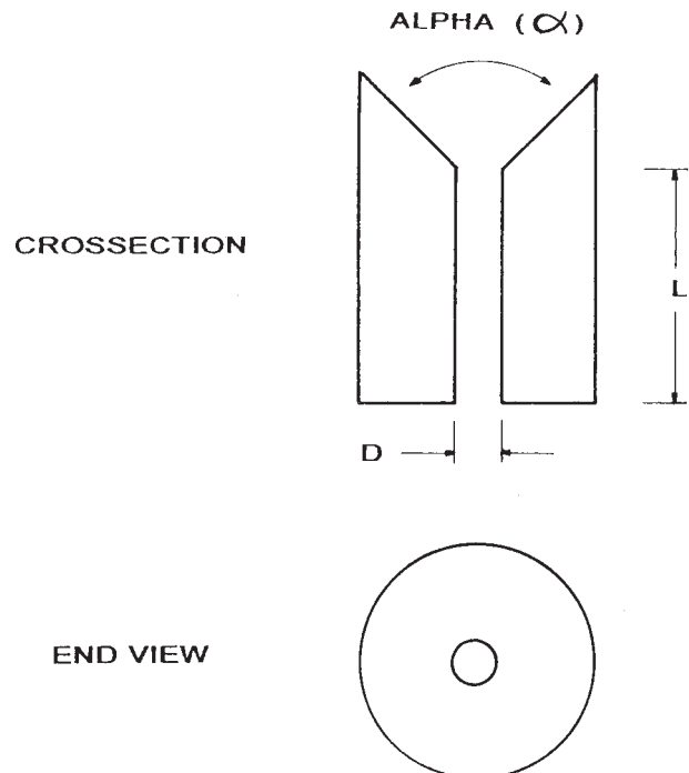
FIG. 2 Rheometer Die
