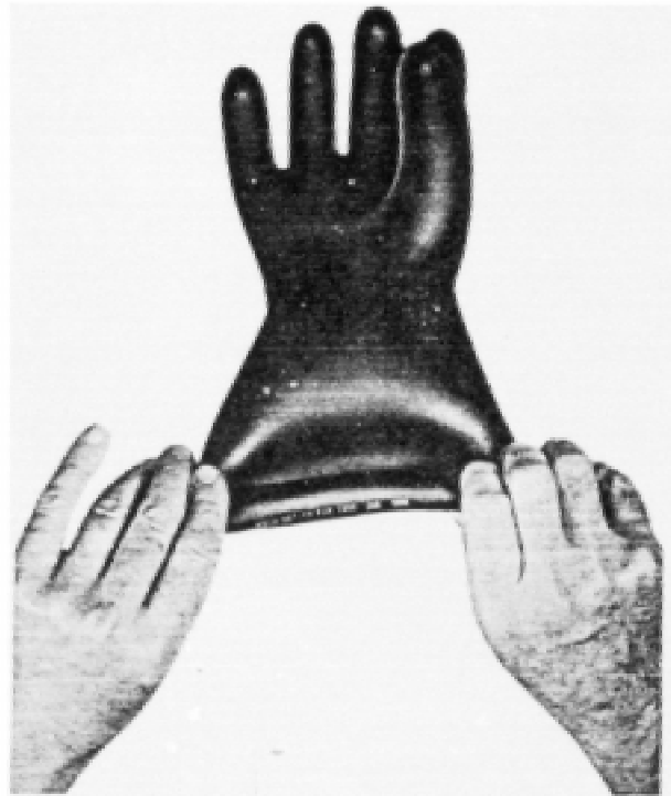
FIG. 31 Stretching
