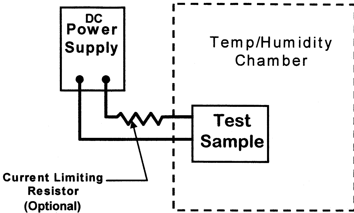
FIG. 1 Test Setup
