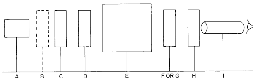
FIG. 1 Polarimeter
