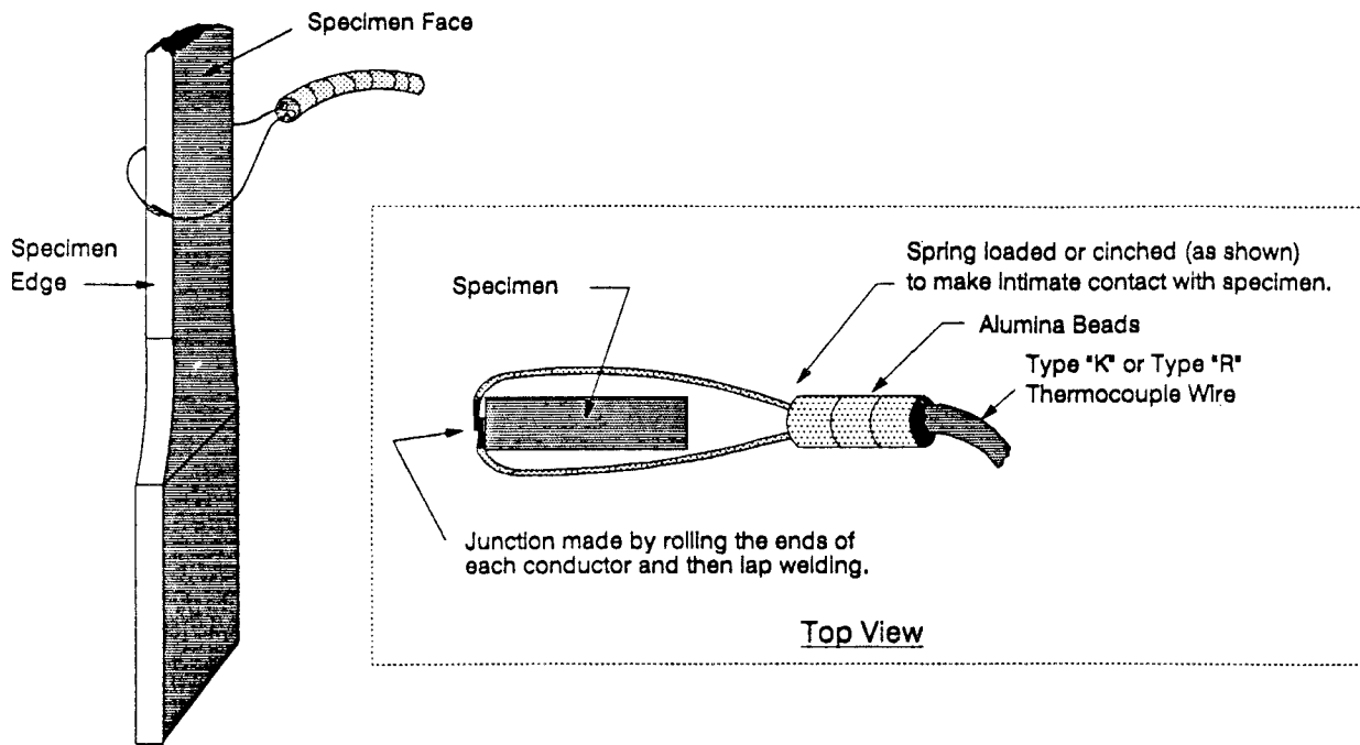
FIG. 6 Wraparound Thermocouple
