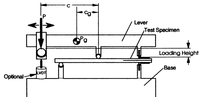
FIG. 1 MMB Apparatus
