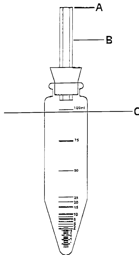
FIG. 1 Apparatus Assembly
